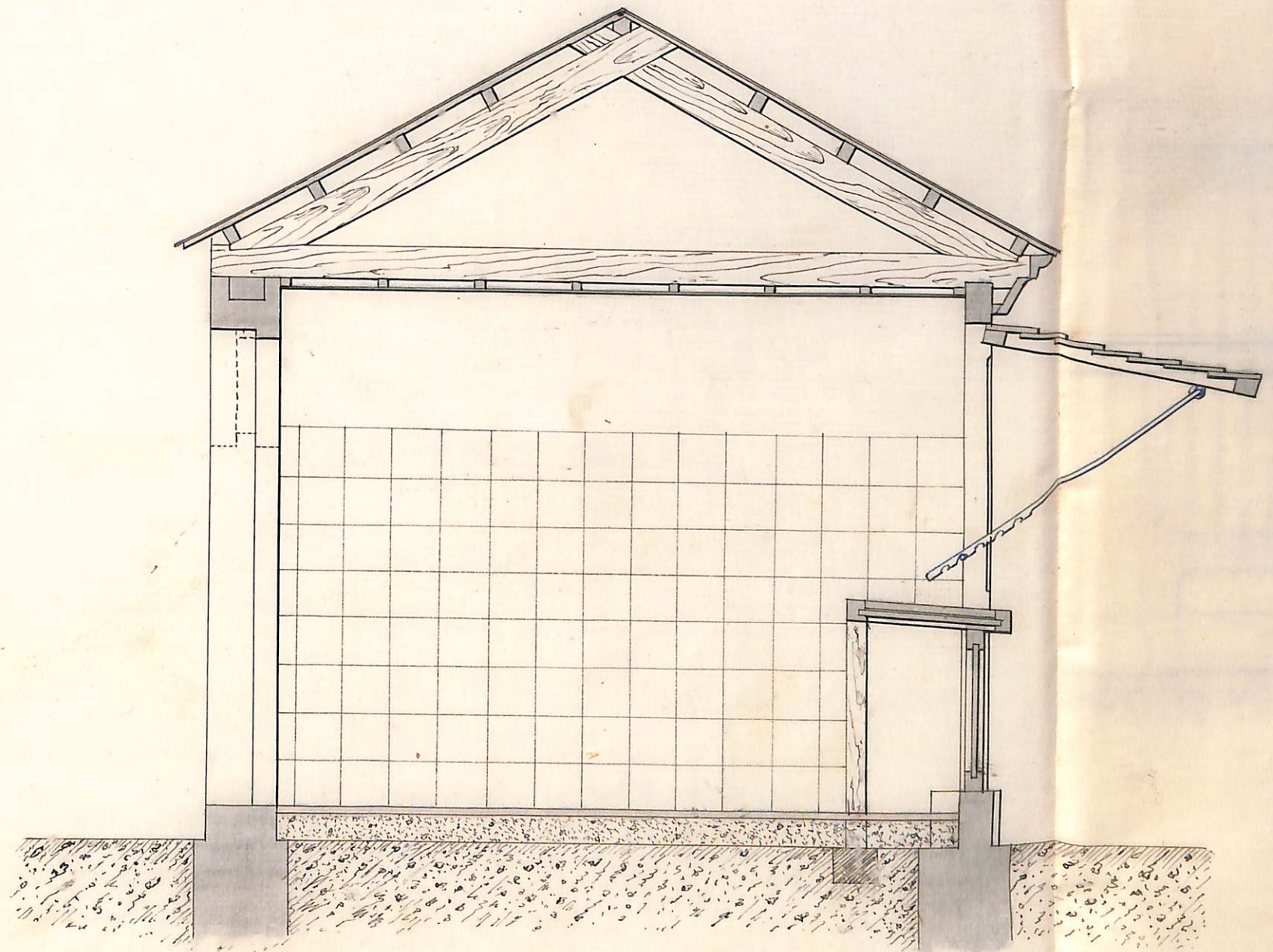
SECCION.
